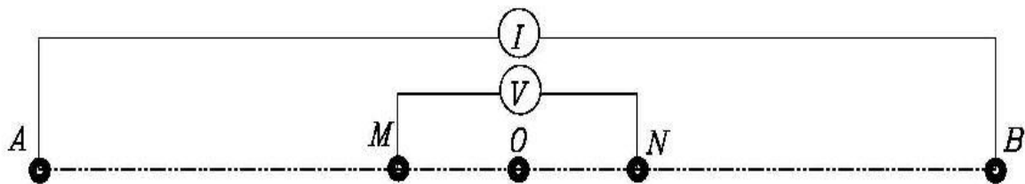
شکل شماره ۳- آرایه شولمبرژه استفاده شده در این مطالعات
