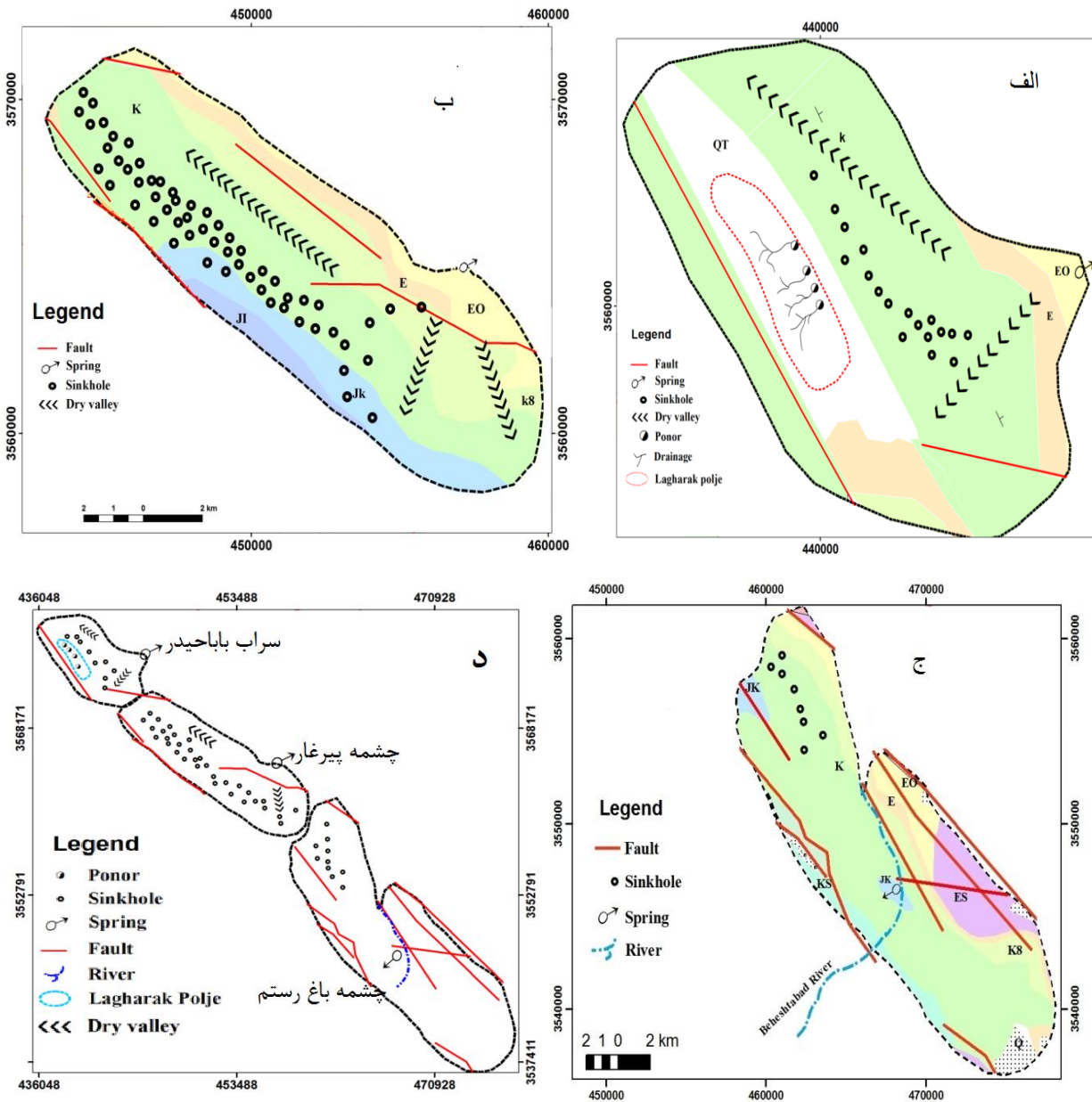
شکل ۶- ارتباط بین ویژگی‌های ژئومورفولوژیکی منطقه با جهت عمومی جریان آب زیرزمینی در تاقدیس سالدوران (الف) سراب باباحیدر (ب) چشمه پیرغار (ج) چشمه باغ رستم (د) موقعیت کلی چشمه‌ها
