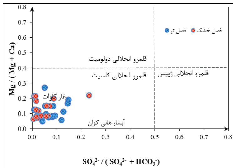
شکل ۶ - موقعیت نمونه‌های منابع آبی مورد مطالعه روی نمودار ترکیبی دو متغیره SO_4^{2-} / (SO_4^{2-} + HCO_3^-) در مقابل Mg / (Mg + Ca) .
