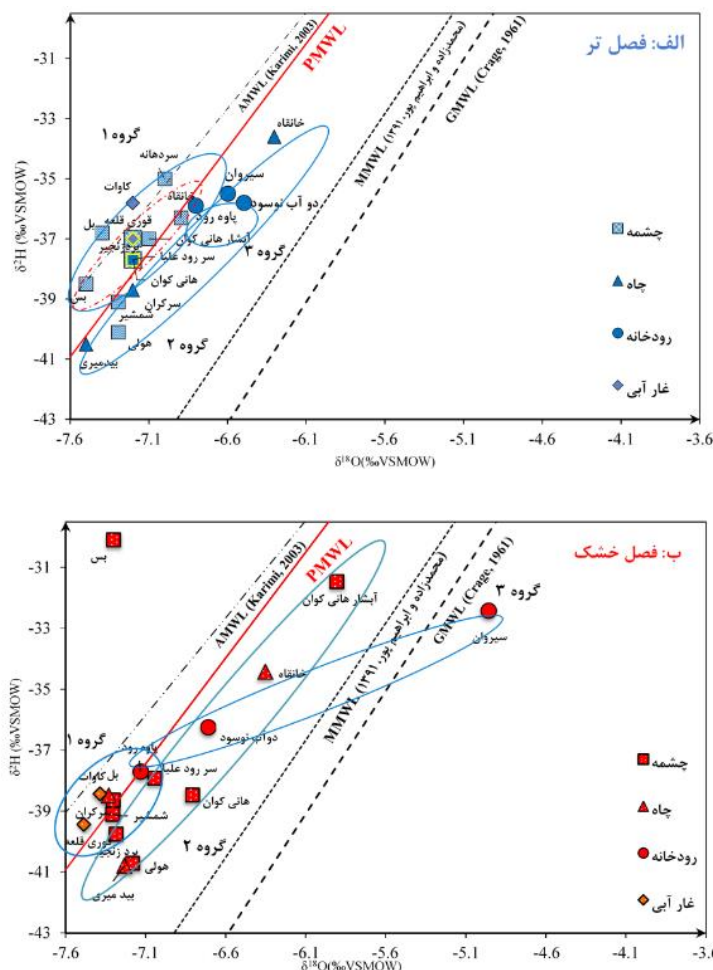
شکل ۸- ترکیب ایزوتوپی منابع آبی پاوه و جوانرود و موقعیت آن‌ها روی دیاگرام \text{H}^2 نسبت به \delta^{18}\text{O} در نمونه‌برداری فصل‌های تر (الف) و خشک (ب)، (محمدزاده، ۱۳۹۵).
