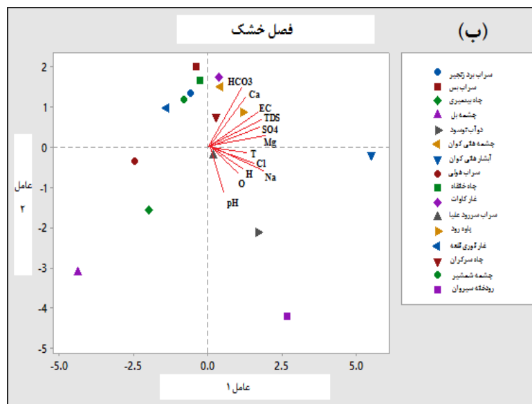
شکل ۷ - طبقه‌بندی منابع محدوده‌های مطالعاتی پاه و جوانرود بر اساس عامل اصلی.
