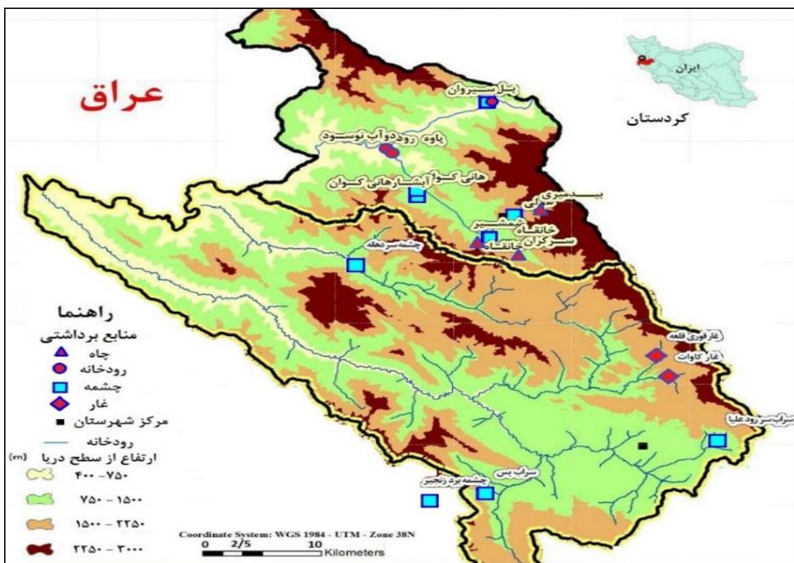
شکل ۱ - نقشه زمین‌شناسی محدوده مطالعاتی پاوه (الف) و جوانرود (ب)، تصویر ماهواره‌ای منطقه و سینک‌هول‌های زاگرس در سازند بیستون (ج)، منابع انتخابی نمونه‌برداری شده در محدوده‌های مطالعاتی پاوه و جوانرود (د).
